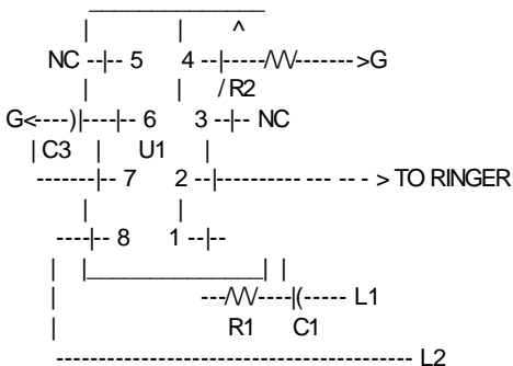
a. Main ringer TTL circuit
