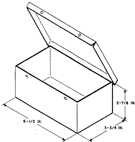
Fig. 5—No. 33 Plastic Goggles Case
