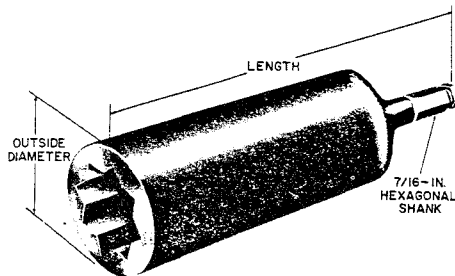
Fig. 4—B Socket
