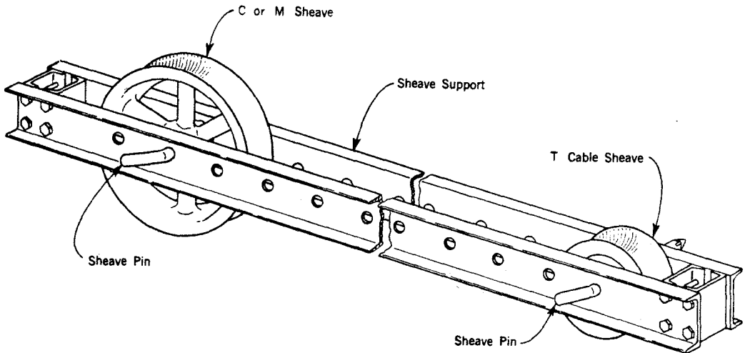
Fig. 1—Pulling Frame
