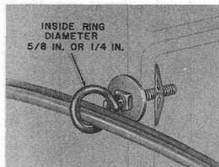
Fig. 2—Toggle Bridle Ring
