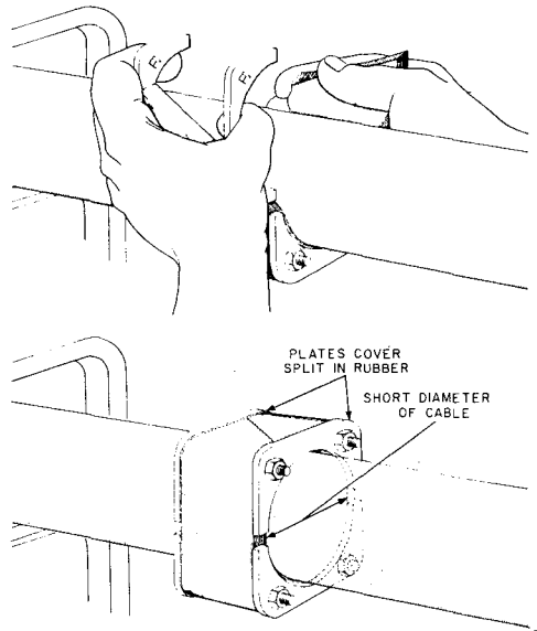
Fig. 4—Placing Split Rubber Conduit Plug on Cable
