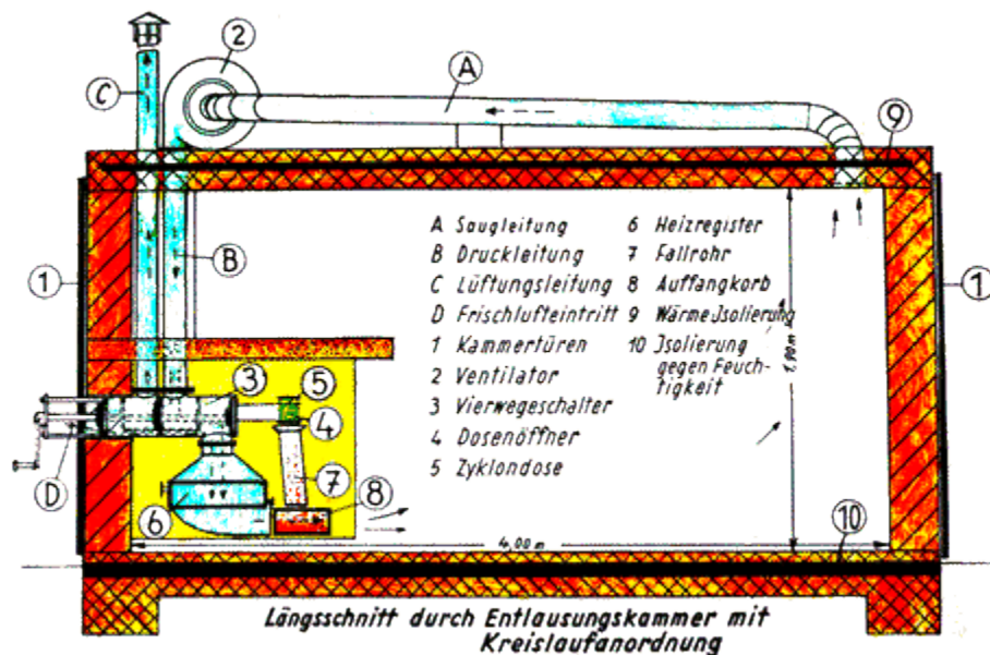
Abb. 26. Längsschnitt durch eine Entlausungskammer mit Kreislaufanordnung
