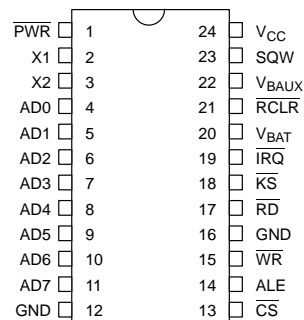
DS17285 24-PIN DIP DS17285S 24-PIN SOIC
