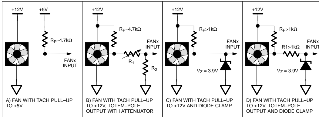
FAN TACHOMETER INPUT OPTIONS Figure 3
